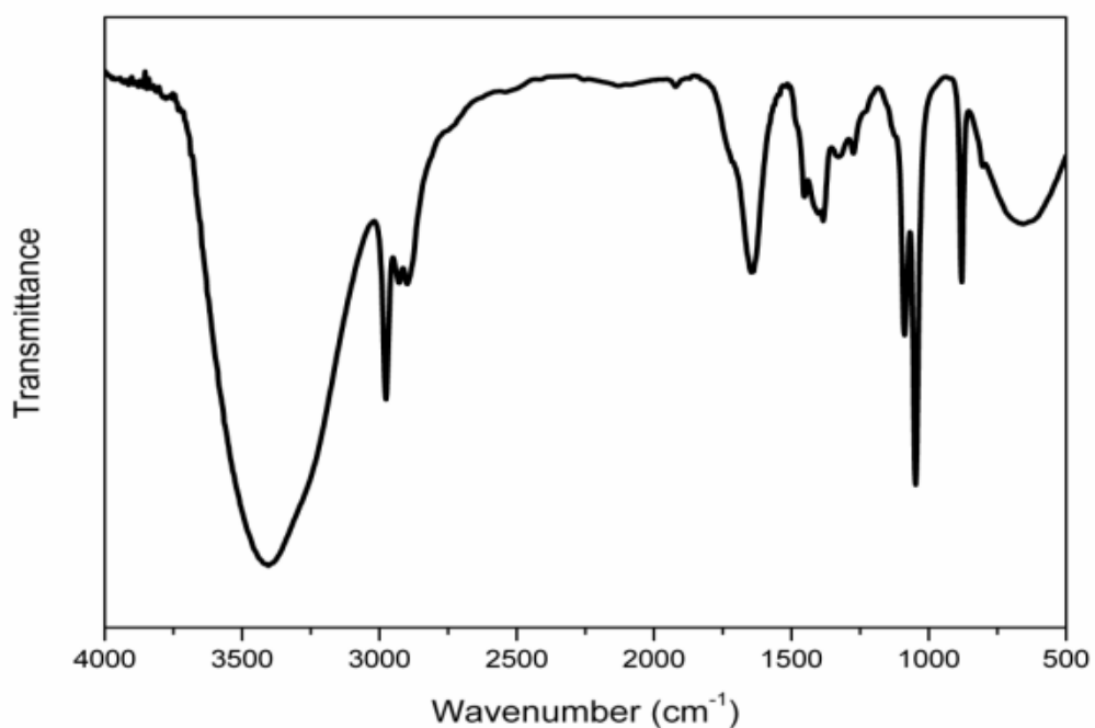
红外光谱图
